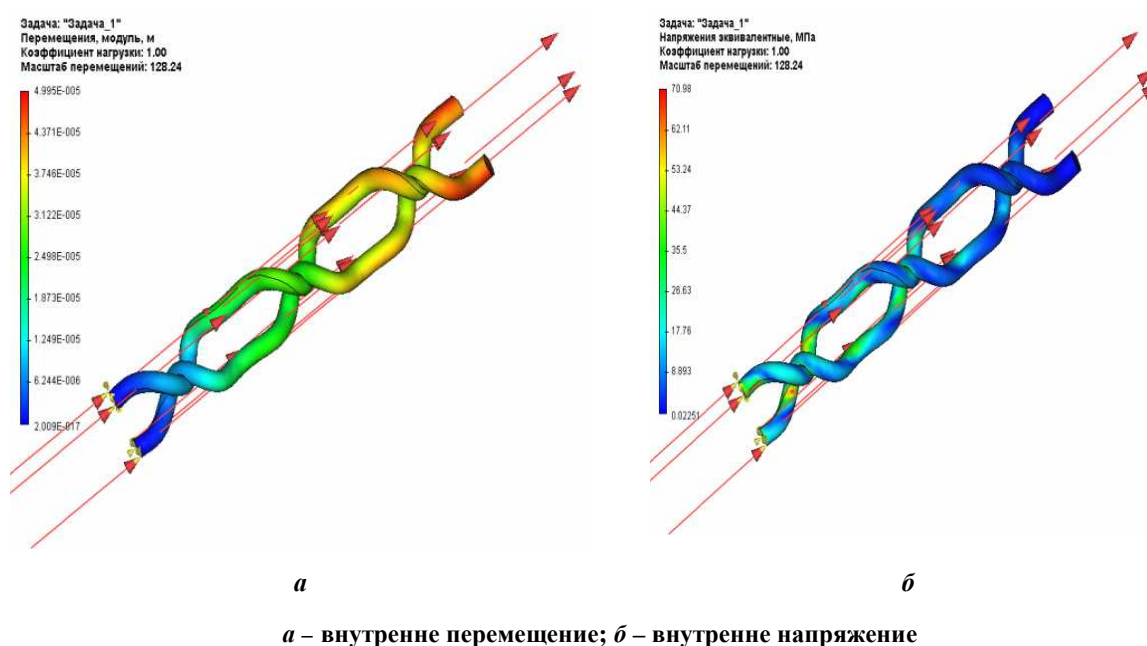
Рисунок 4. – Деформации напряжения растяжения, испытываемые моделью заданного профиля
