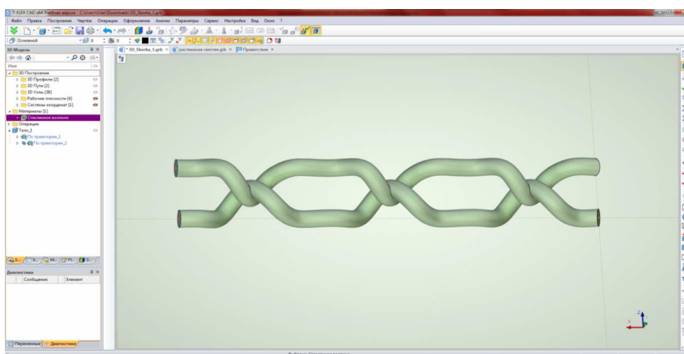
Рисунок 3. – Рабочее окно программы T-FLEX CAD с построенной 3D-моделью выбранного профиля стеклопластиковой арматуры
